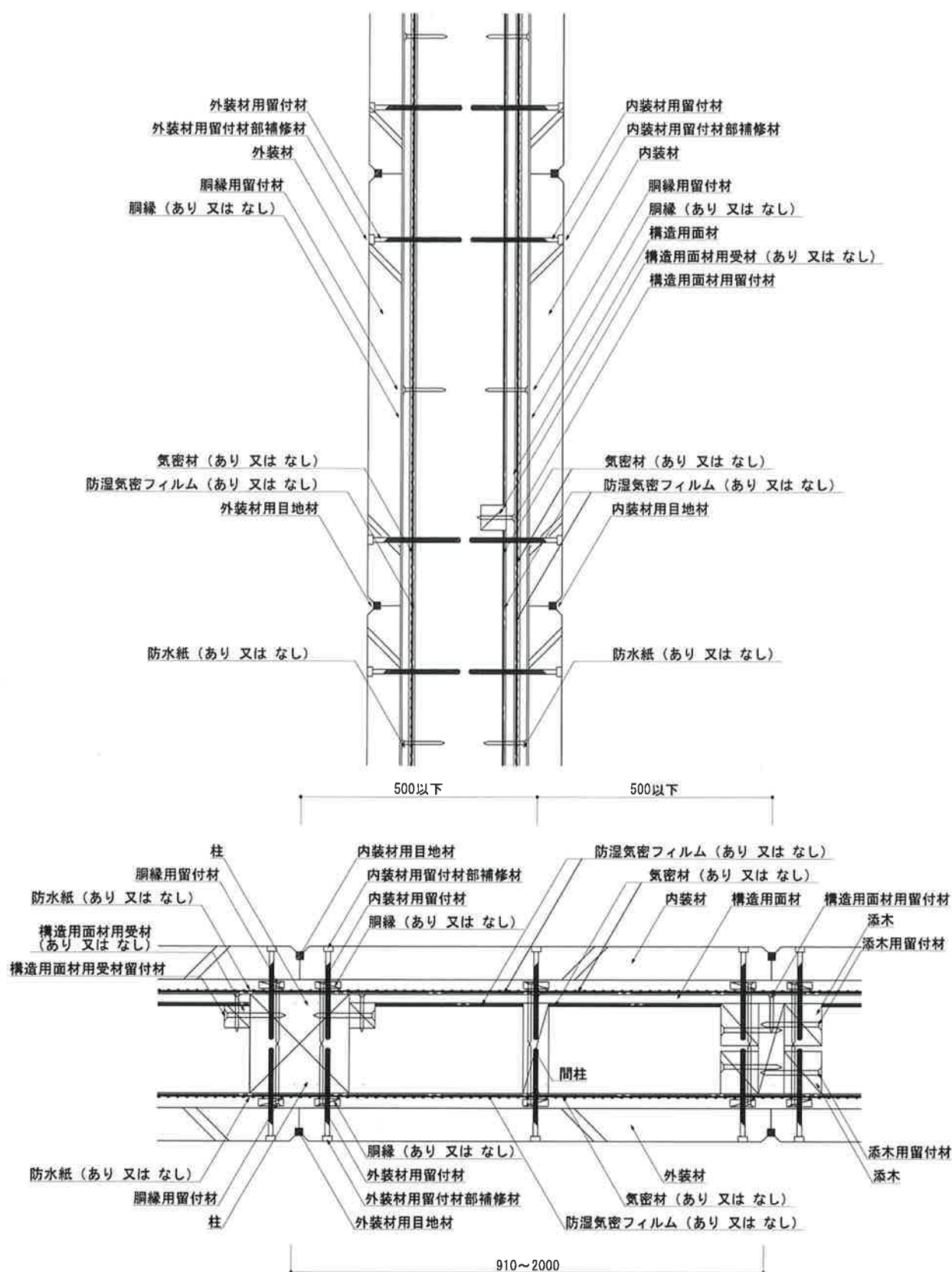
図4 構造説明図 (水平垂直断面詳細図・屋外側構造用面材なし／屋内側構造用面材真壁)
