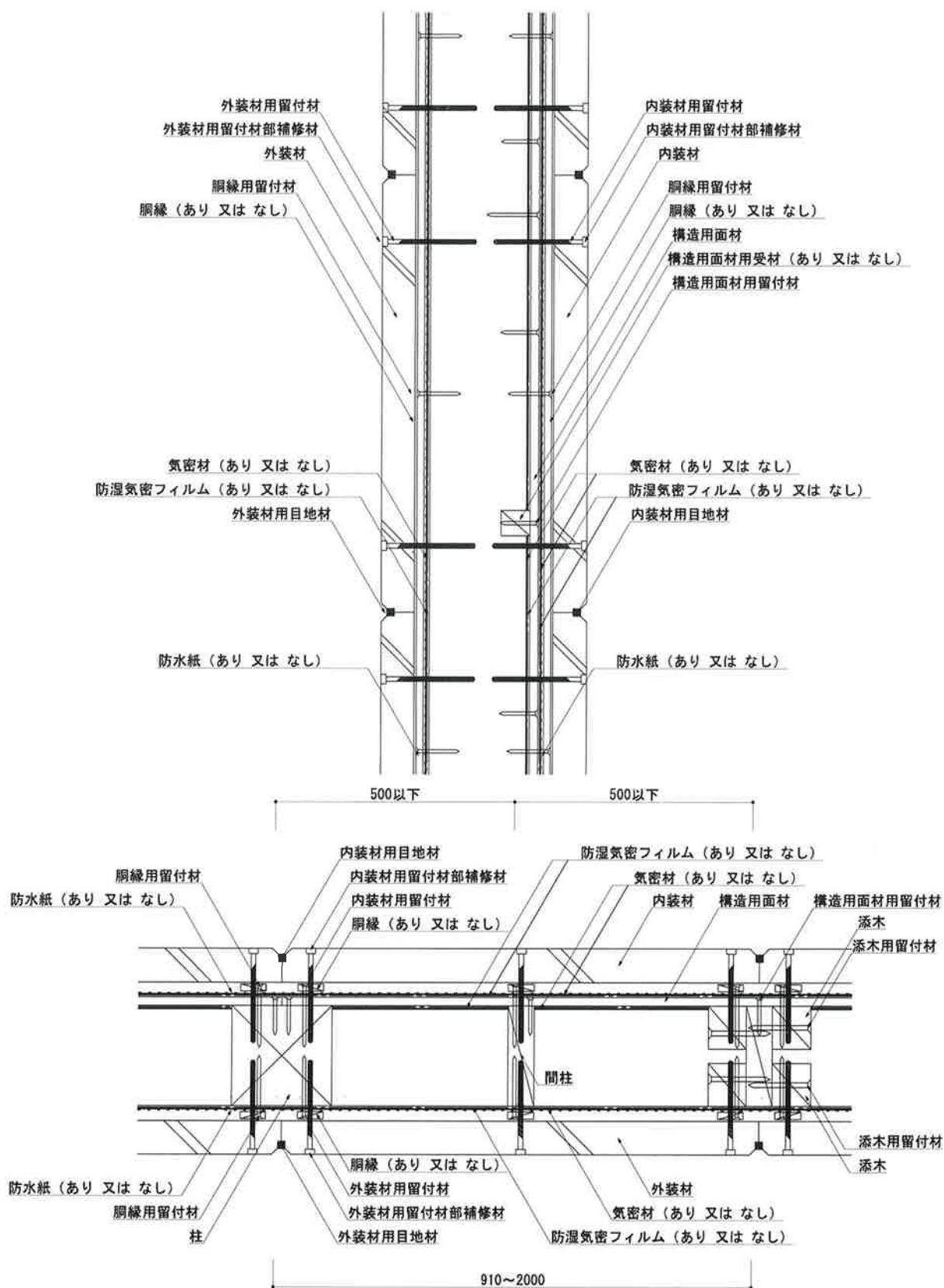
図2 構造説明図 (水平垂直断面詳細図・屋外側構造用面材なし／屋内側構造用面材大壁)
